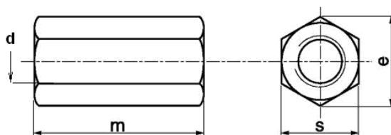
Гайка удължена, DIN 6334, поцинкована, клас на якост 6
